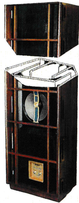
(リヤロード/カーブホーン構造図)
